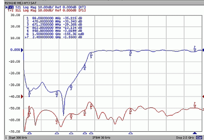
Charakterystyka toru TV. Kolor czerwony - dopasowanie, kolor niebieski - tłumienie
