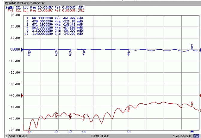
Charakterystyka toru SAT-2 (kanał zwrotny). Kolor czerwony - dopasowanie, kolor niebieski - tłumienie.
